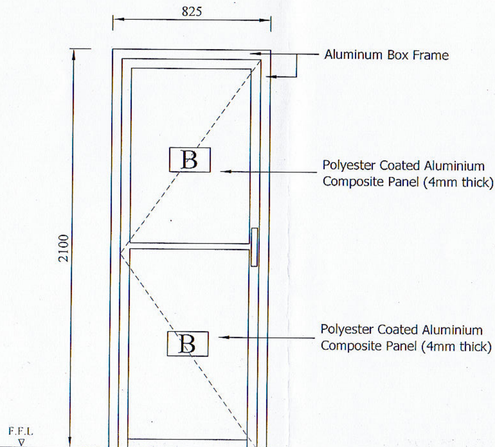
D20(TOILET DOOR)
